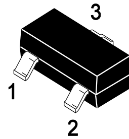
1.GND 2.VOUT 3.VIN
